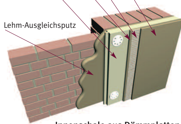
Innenschale aus Dämmplatten
